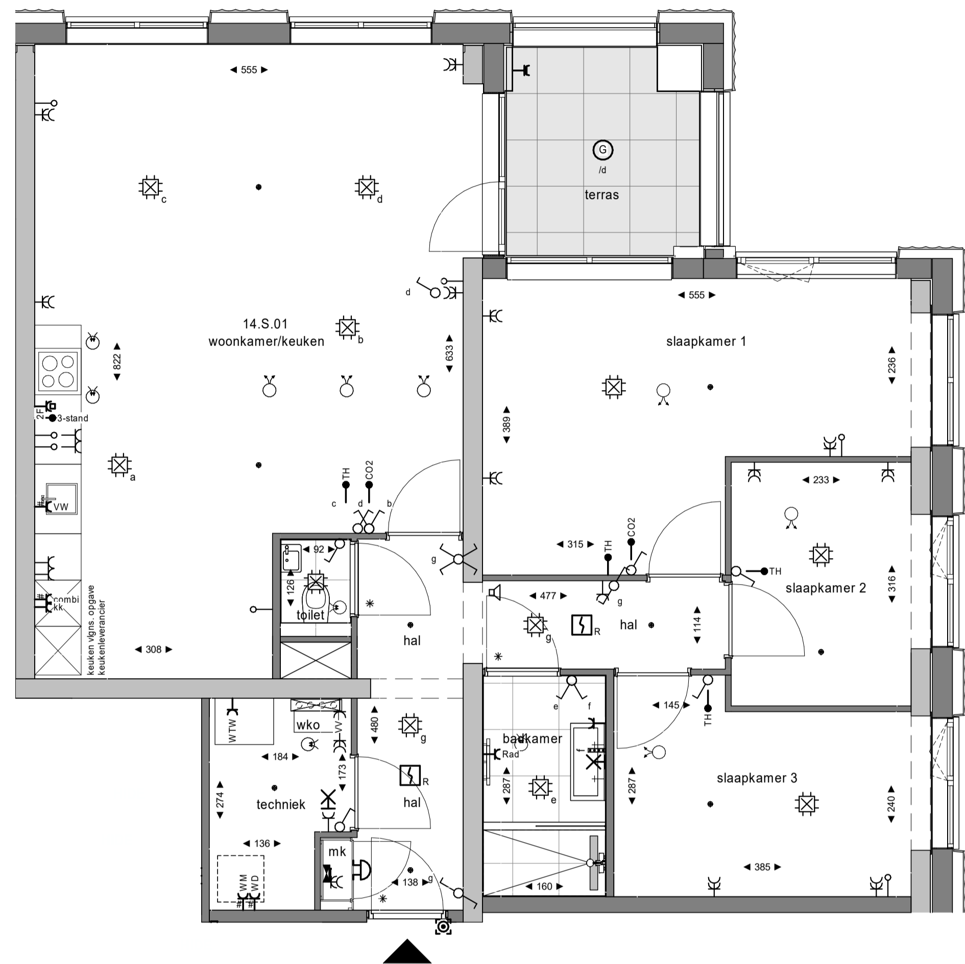
plattegrond 1 : 50 14e verdieping
